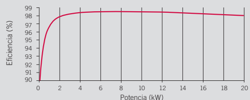
Rendimiento INGECON® SUN 20TL Vdc = 600 V
