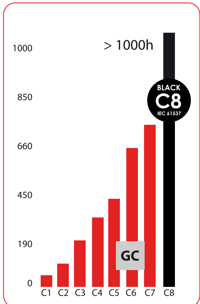
Duración (h) ensayo Camara niebla salina, según ASTM-B117 Duração (h) Teste Camara de nuvem salina, conforme ASTM-B117
